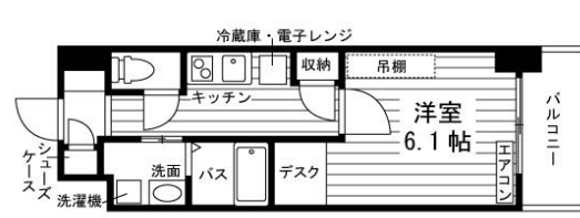
Fタイプ 1K (25.2㎡)
